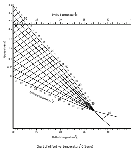
上図：具体的な風速が体感温度にどのような影響を及ぼすかを示した米国の研究
