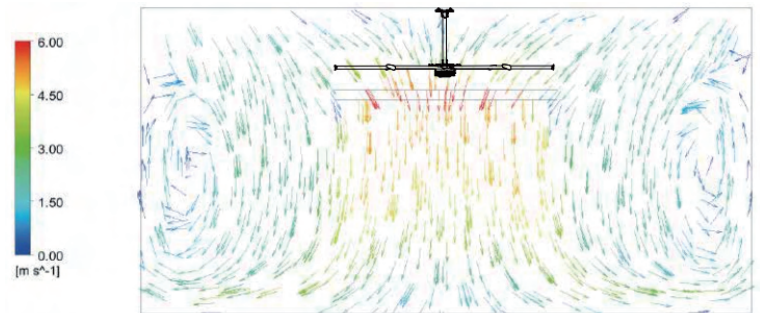
HVLSファン設置高さ:7m 気流層:3m 測定地点高さ:1.5m
