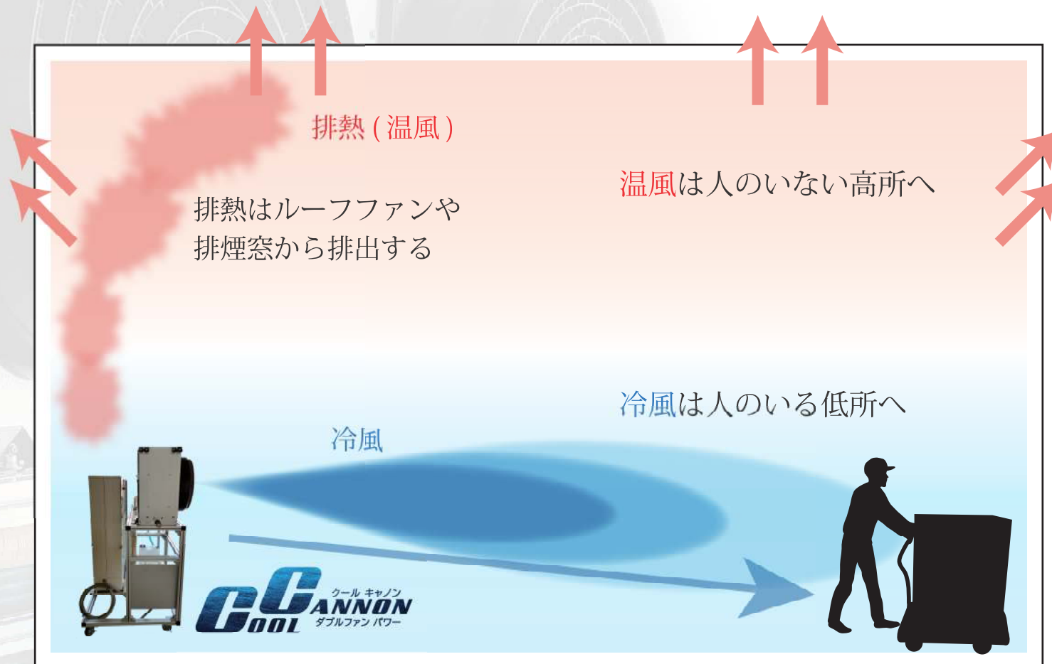
■設置イメージ(断面図)
